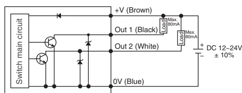
NPN Output
